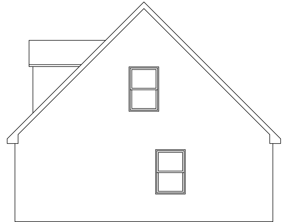
RIGHT ELEVATION
